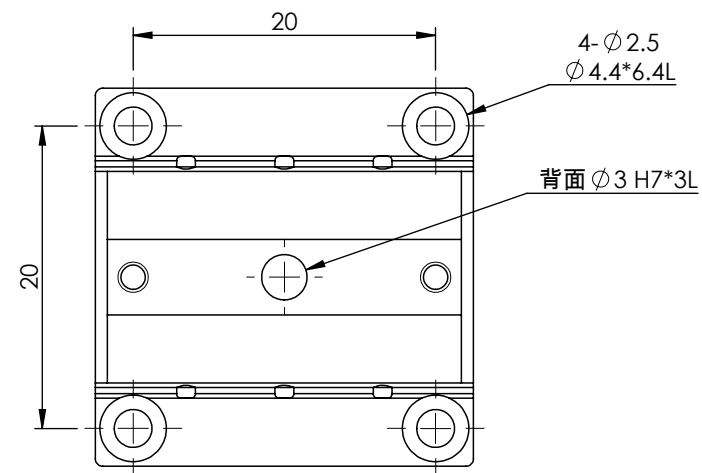
MX(Y)25-S-28系列 底座安裝孔尺寸
