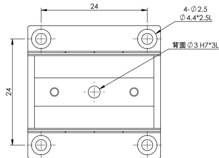
MX(Y)30-S-28系列 底座安裝孔尺寸
