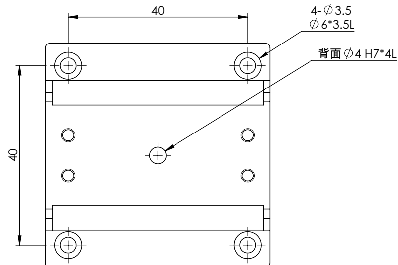
MX(Y)50-S-28系列 底座安裝孔尺寸
