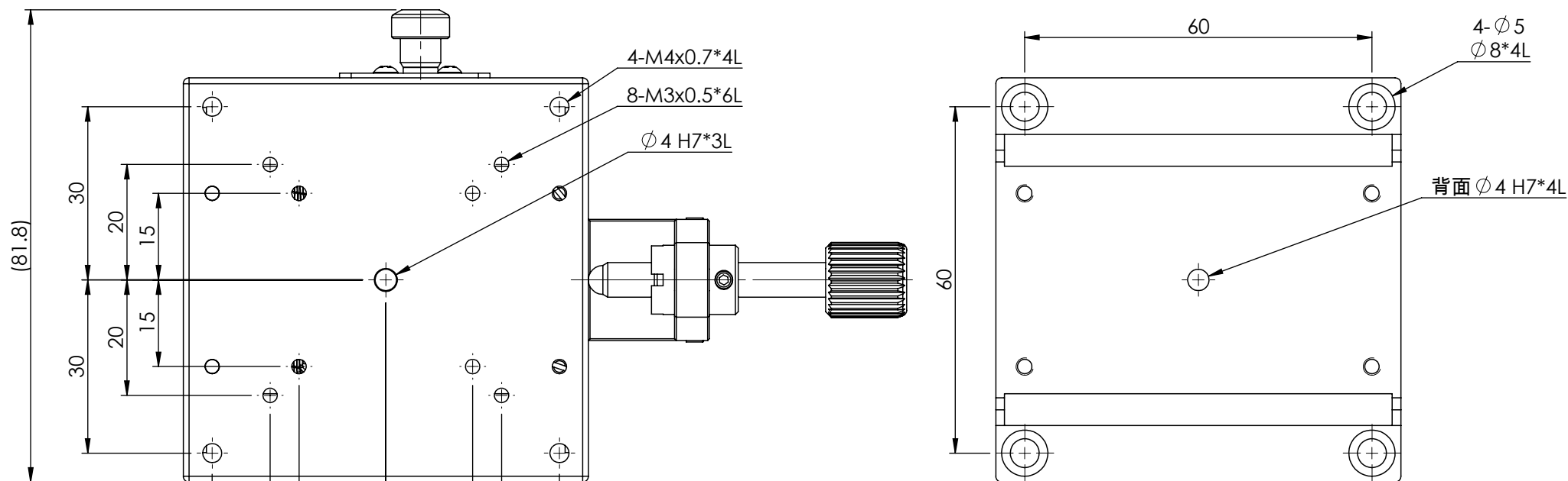
MX(Y)70-S-28系列 底座安裝孔尺寸
