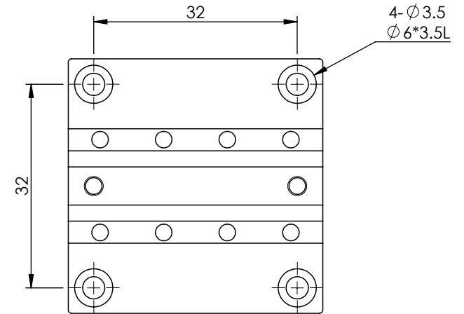
底部安裝孔尺寸
