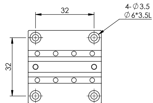
底部安裝孔尺寸
