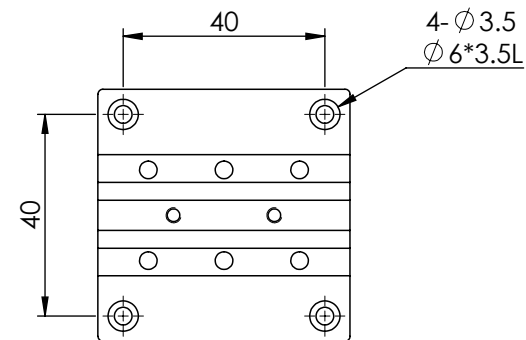
底部安裝孔尺寸
