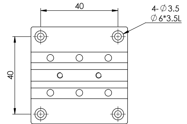
底部安裝孔尺寸
