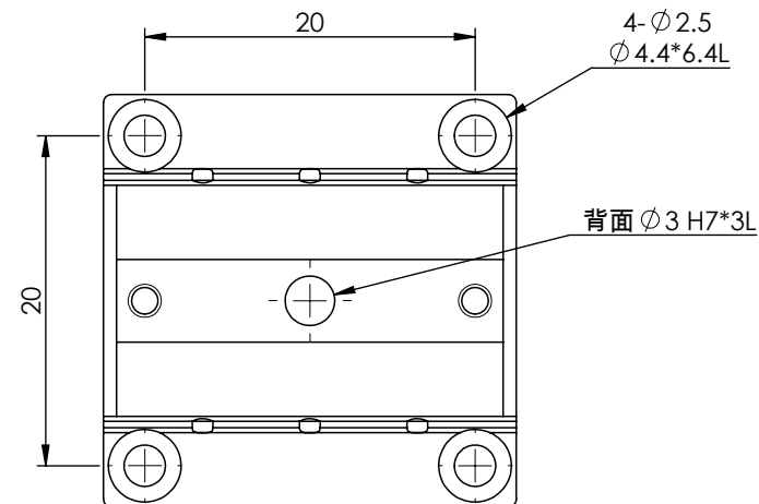
MX(Y)25-S系列 底座安裝孔尺寸
