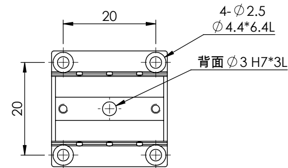
底部安裝孔尺寸
