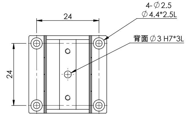
底部安裝孔尺寸
