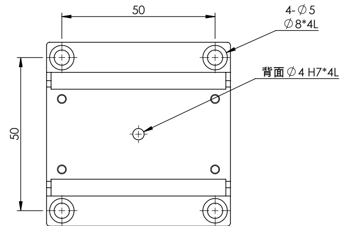
底部安裝孔尺寸
