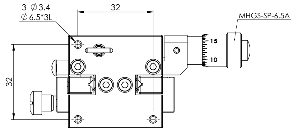
底部安裝孔尺寸
