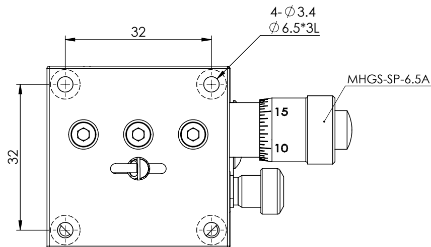
底部安裝孔尺寸
