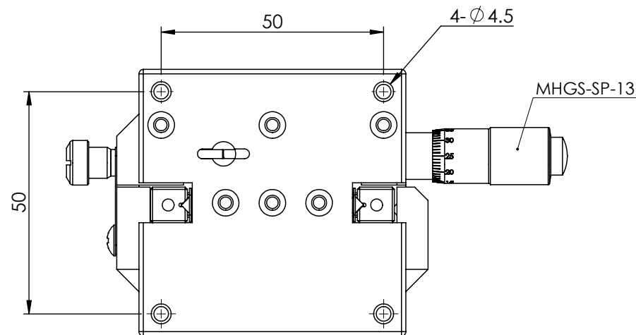
底部安裝孔尺寸
