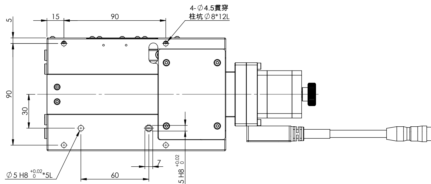
底部安裝孔
